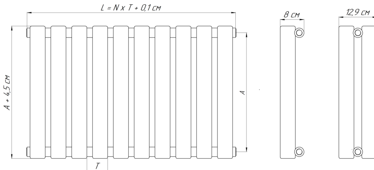
Рис. 1 Радиатор «Гармония», где: А – межцентровый размер, см; Т – шаг (Т = 7 см); N – количество секций; L – габаритная длина, см.
